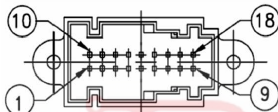
◇ 18 PIN AMP CONNECTOR : (AMP 953264-1,WHITE)
